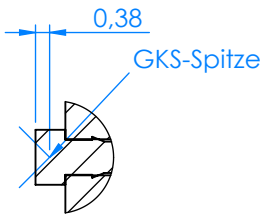
DETAIL X MAßSTAB 5 : 1
