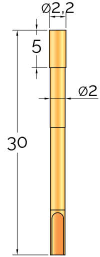
CR 112 - 3G8 wire wrap
