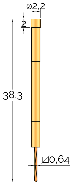
CR 112 - 3E2 wire wrap
