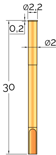
CR 112 - 3 wire wrap
