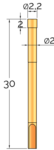
CR 112 - 3E5 wire wrap
