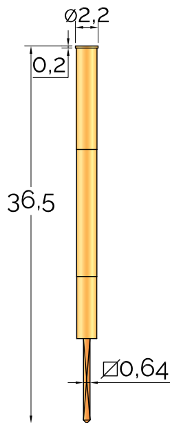
CR 112 - 3 wire wrap
