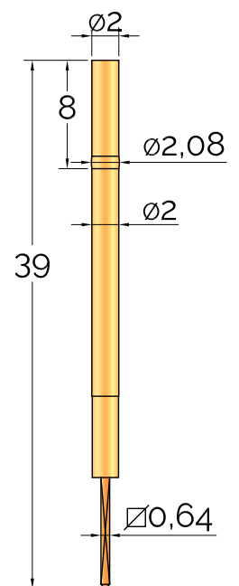
CR 112 - 3G8 wire wrap
